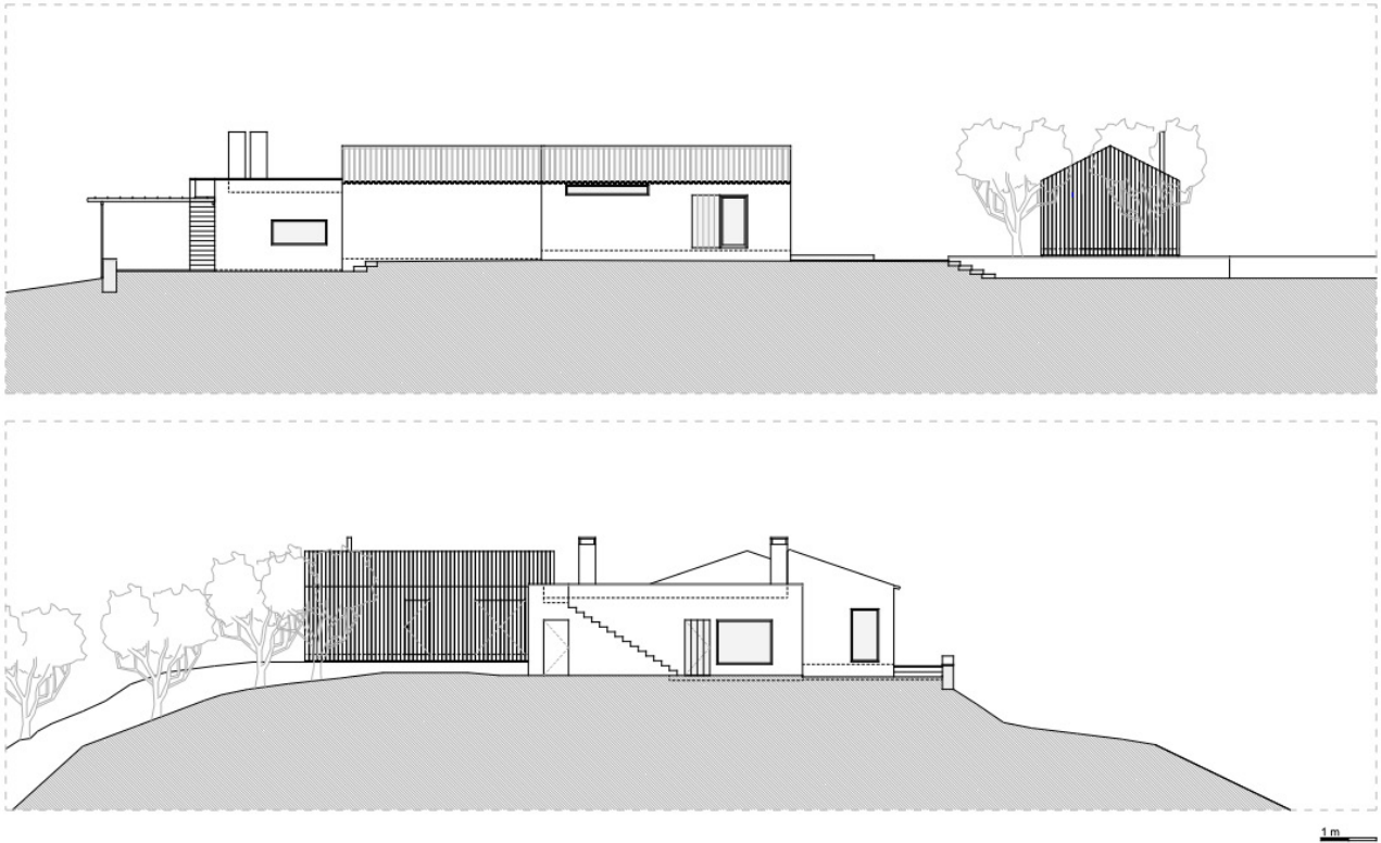
Alçados Sudeste e Noroeste
