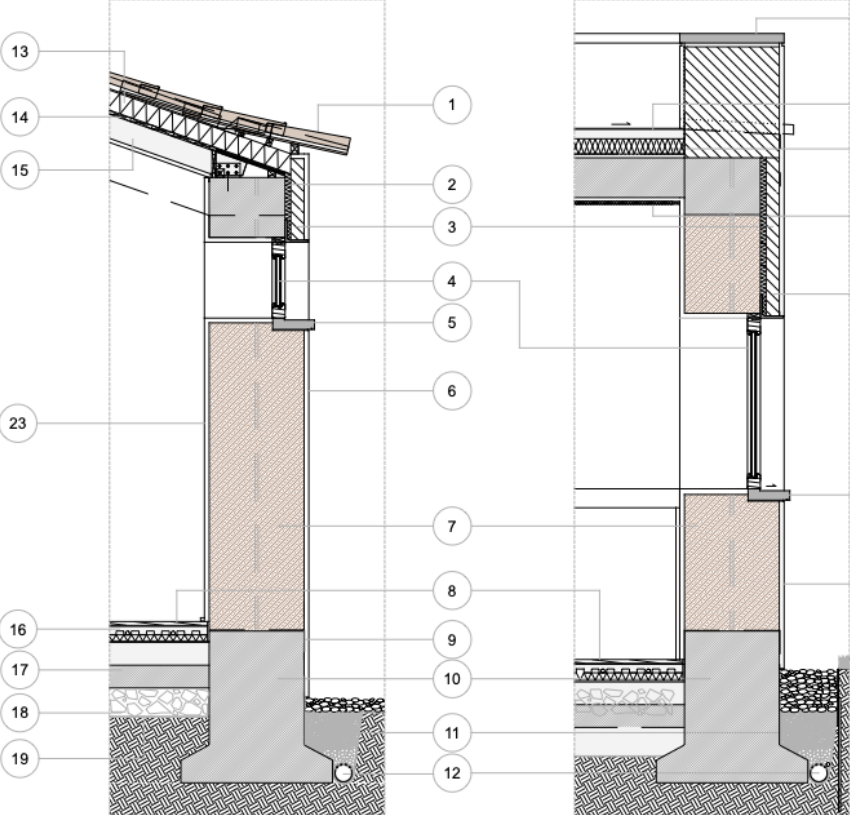
Corte construtivo
