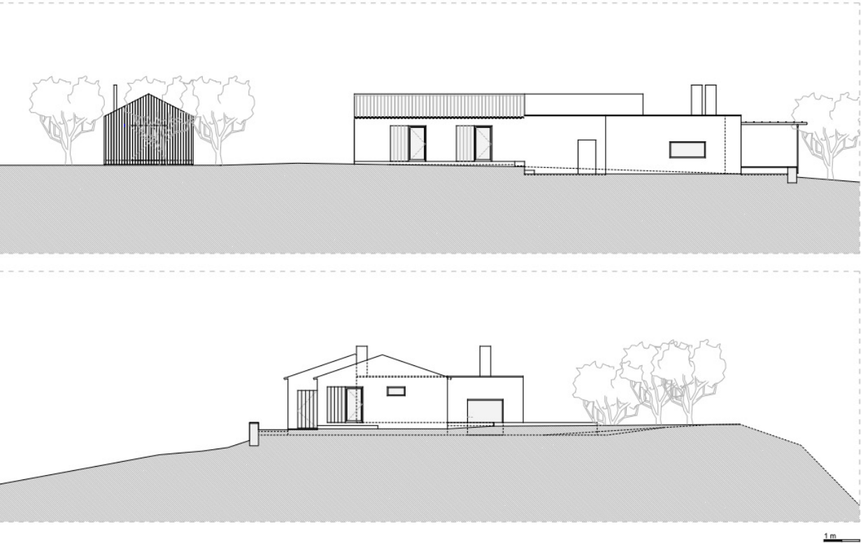
Alçados Nordeste e Sudoeste
